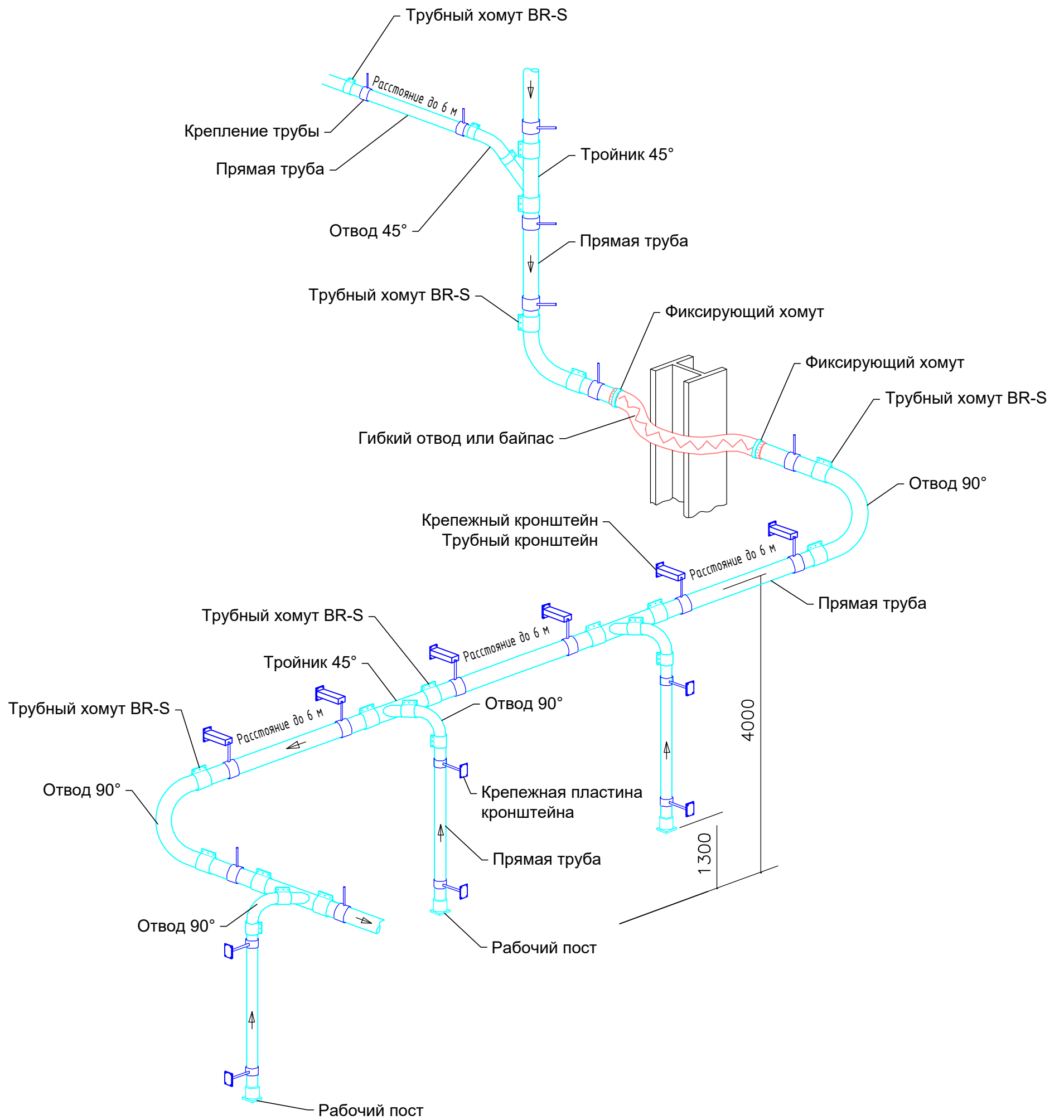
Элементы крепления трубопровода
